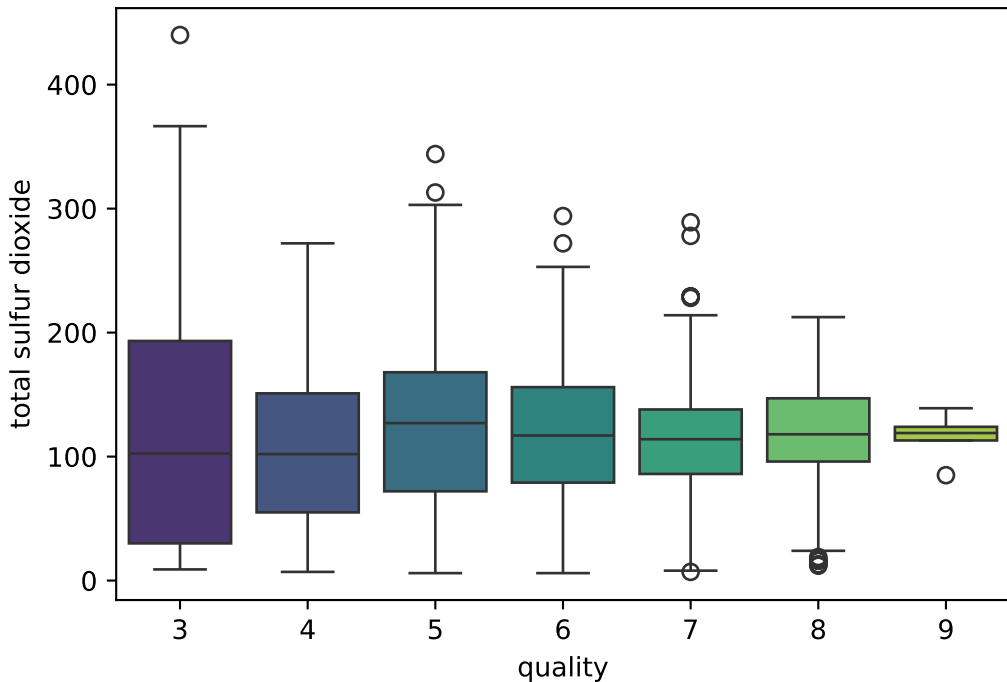
Distribuição Condicional - total sulfur dioxide
